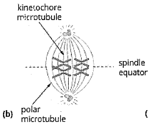
Metaphase I
