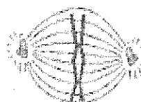
Metaphase II
