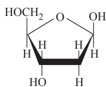
deoxyribose
