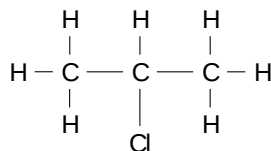
B 2-chloropropane
