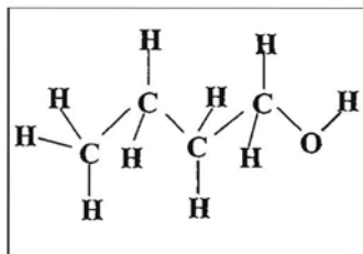
Butan-1-ol
