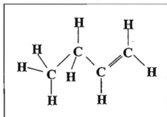
But-1-ene
