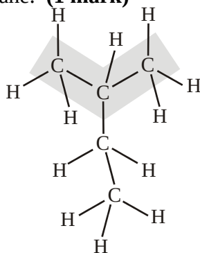
2-ethylpropane
